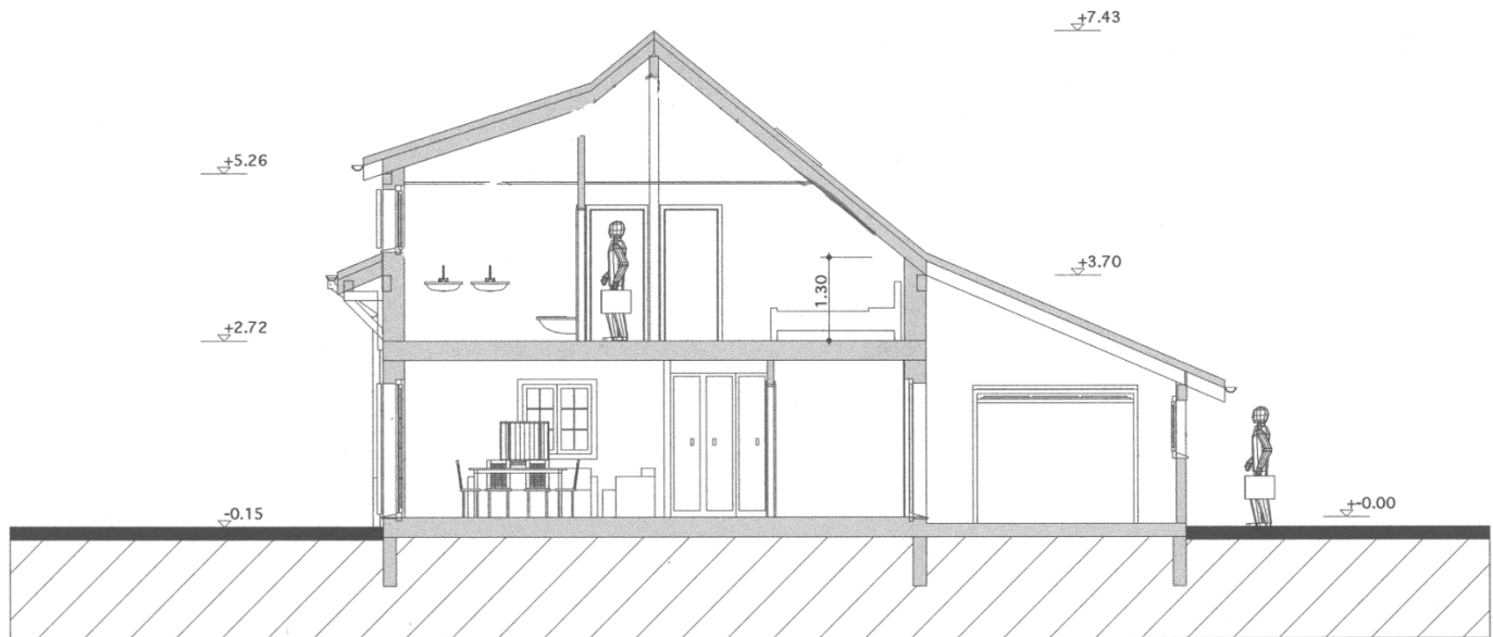
Coupe A-A
